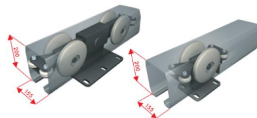
Kraftig bærebjelke og hjulføring.
